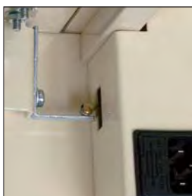
Interrupteur fin de course coupant l'alimentation de l'écran en position rabattue.
